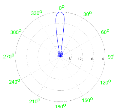
Vertikální vyzařovací diagram
