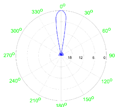
Vertikální vyzářovací diagram
